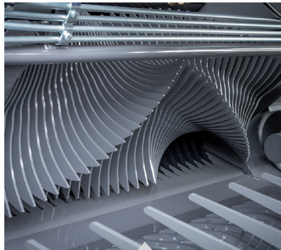
Snijrotor met 25 messen.
