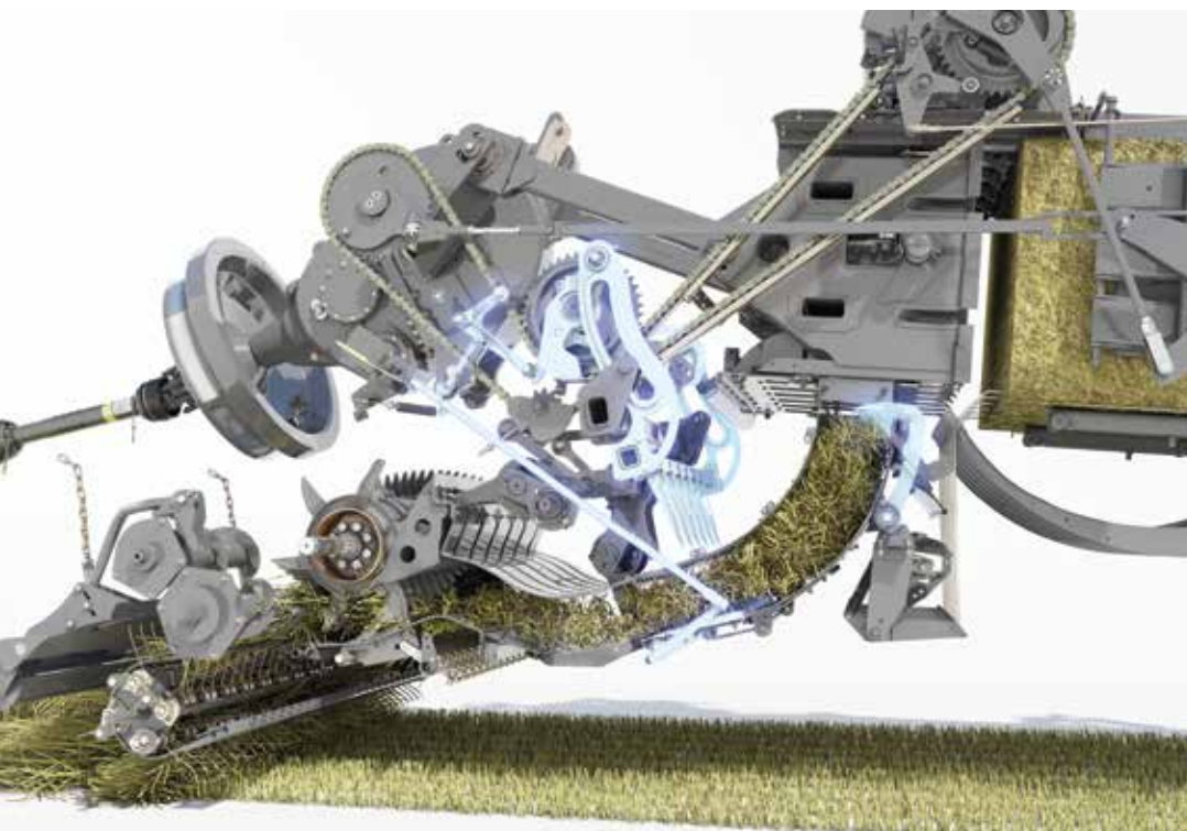
Voorperskamer - vullen.
