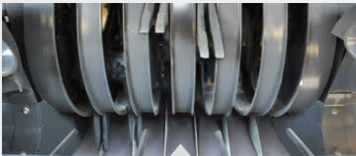
Pakker snijinrichting voor MF 2240** en MF 2250.
